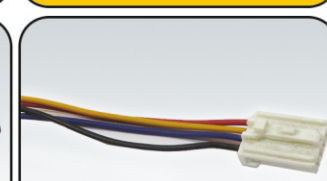
سوکت ساعت سمند
