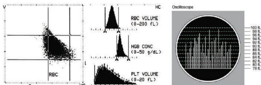
شکل ۱-۹. از راست به چپ شامل نمودار اسیلوگرام، هیستوگرام و سیتوگرام مربوط به اریتروسیت‌های مورد شمارش در یک دستگاه سل کانتتر بر پایه امپدانس و پراکنش نوری
