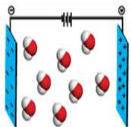
شکل ۱۷- جهت گیری مولکول های آب در میدان الکتریک
