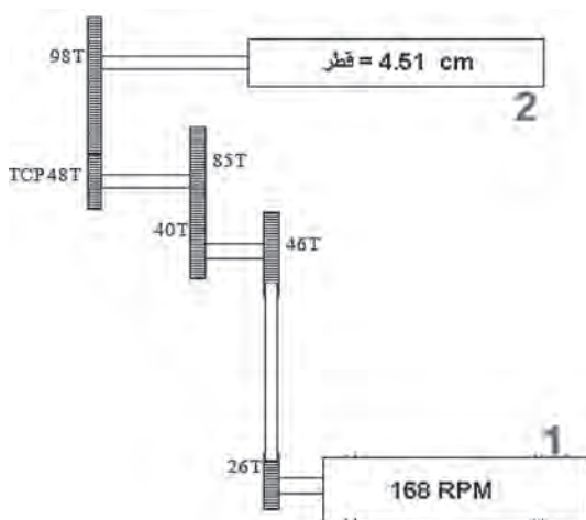
شکل ۱۹- چرخ دنده‌ها در انتقال نیرو
