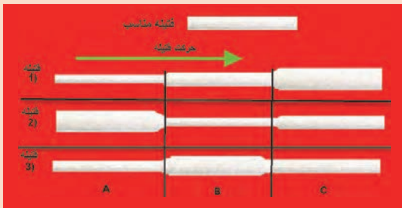
شکل ۱۸- چند نمونه فتیله ورودی به اتولولر
