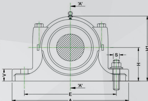
نمای روبرو
