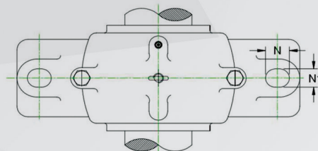
نمای بالا
