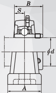
نمای کنار
