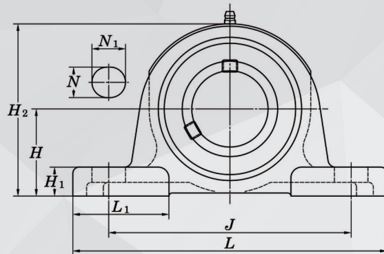
نمای روبرو
