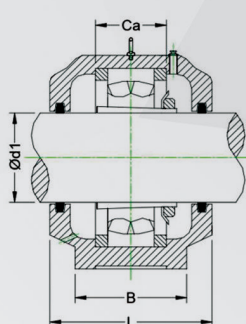
نمای AA
