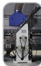
ایستگاه سر و ته زن ایستگاه فرز بالا و پایین
