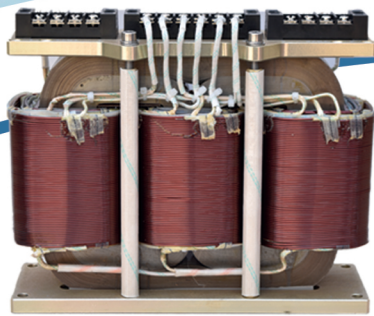
5KVA-400HZ
