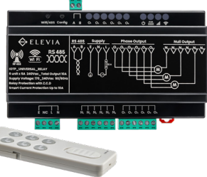
* MC-1812 مازول پرده هوشمند
