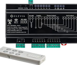
* MR-1811 مازول ۹ رله هوشمند
