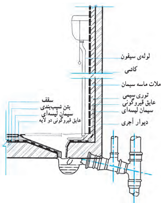
شکل ۳-۲۳۰ مراحل اولیه نصب کاسه توالت ایرانی
