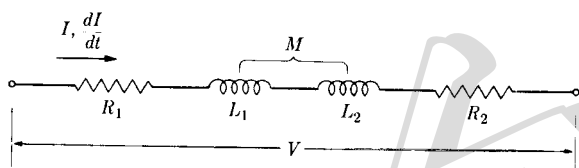
شکل ۳۰۱۱ اتصال متوالی دو القاگر
