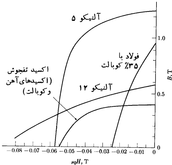
شکل ۹.۹ منحنیهای پسماند برای مواد آهنربای دائم. (توجه کنید که H به جای \mu_0 H در روی محور افقی رسم شده است.)
