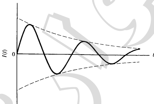
شکل ۵۰۱۳ پاسخ گذرای يك مدار RLC .
