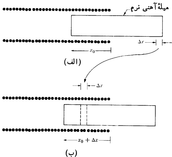
شکل ۱۰.۱۲ نیروی وارد بر میله‌ای از آهن نرم که وارد یک سیم‌لوله شده است (با استفاده از روش انرژی). H-M
