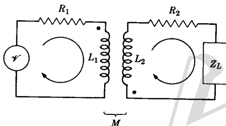
شکل ۱۲.۱۳ مبدل.
