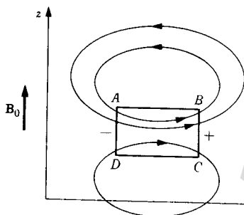
شکل ۸.۱۴ قسمت ABCD ی پلاسما در جهت مثبت z حرکت می کند. جریانهای که به وجود می آیند به صورت طرحواره رسم شده اند.
