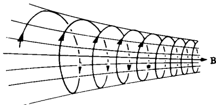
شکل ۴.۱۴ ذره در مسیری مارپیچی که مرتباً تنگتر و فشرده‌تر می‌شود می‌چرخد و سرانجام منعکس شود. H--
