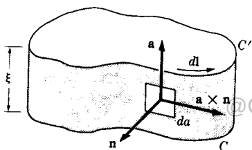
شکل ۶.۱ حجمی که در اثر تغییر مکان منحنی C در راستای بردار یکه عمودش، \mathbf{a} ، به وجود می‌آید.
