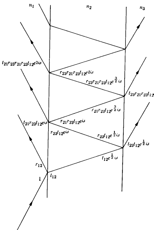
شکل ۸.۱۸ انعکاس و انتقال چندگانه یک پرتو فرودی، بادامنه واحد. هر یک از دامن‌ها با ضرایب فرنی و تأخیر فاز \beta مشخص شده است.
