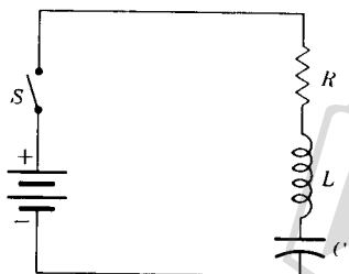
شکل ۴۰۱۳ پاسخ گذرای يك مدار RLC . نمودار مدار.
