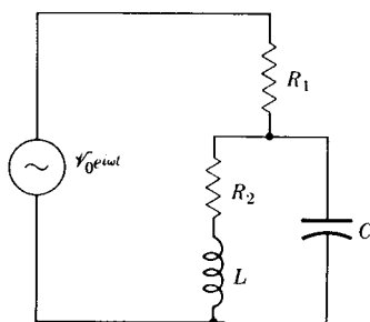
شکل ۶.۱۳ یک نمونه از مدار ac.
