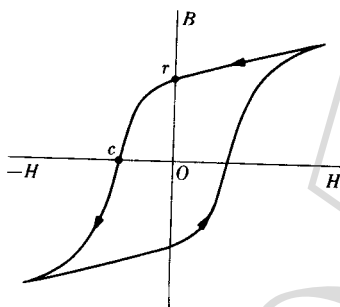
شکل ۶.۹ حلقهٔ پسماند نمونه برای یک مادهٔ فرومغناطیسی.
