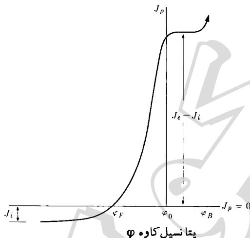
شکل ۹.۱۴ مشخصه جریان - ولتاژ کاوه‌ای که داخل پلاسما شده است. \phi_0 پتانسیل پلاسماست.
