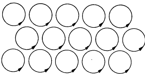
شکل ۱۰۹ تصویر ساده‌ای از ماده مغناطیسی که از جریانهای حلقه‌ای اتمی هم‌جهت تشکیل شده است.
