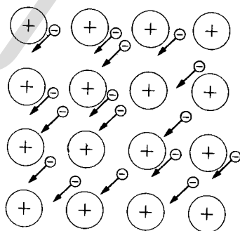
شکل ۱.۷ نمودار طرح‌واره حرکت الکترون‌های رسانش در فلزات.
