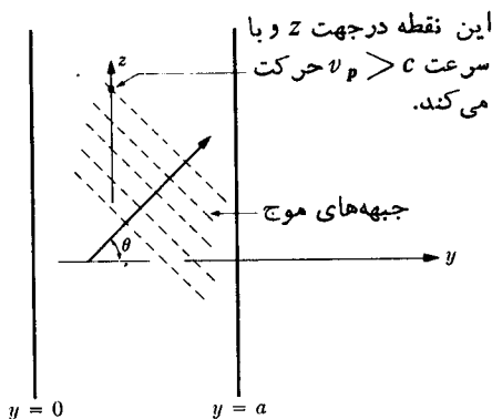
شکل ۱۱.۱۸ جزئیات حرکت جبهه‌های موج در افتخار انتشار موج بین صفحات رسانا.
