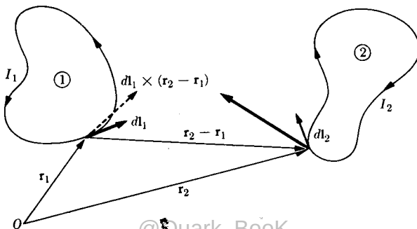
شکل ۳.۸ برهم کنش مغناطیسی دو مدار جریان.
