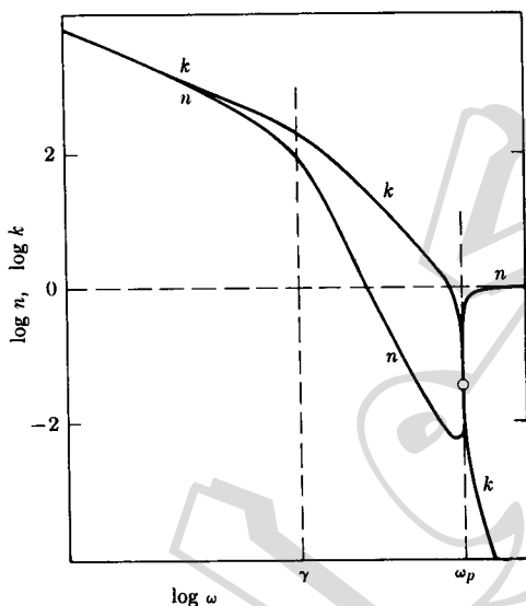
شکل ۶.۱۹ نمودار ثابتهای اپتیکی بارهای آزاد بر حسب فرکانس در مقیاس \log - \log ، با \log \gamma / \omega_p = ۰.۰۰۴ در قسمت اعظم گستره فرکانس تقریبهای قانون توان معتبر است.
