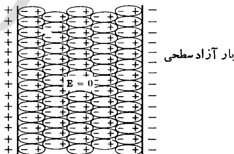
شکل ۵.۵ يك قطعه ماده فروالكتريك قطبیده.
