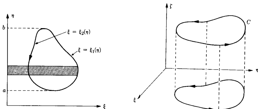
شکل ۲.۸ محاسبه انتگرال \oint \xi d\eta
