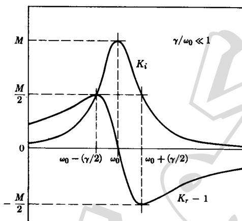
شکل ۳.۱۹ ثابتهای دیالکتریک برای خط باریکی در \omega_0 . (میدافرکانس در فاصله دور در سمت چپ واقع است). برای خط ضعیفی با M \ll 1 ، مقدار n-1 و k به ترتیب درست برابر با نصف K_i و K_r - 1 هستند.
