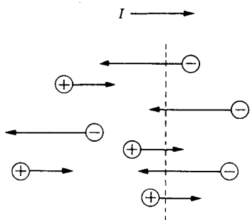
شکل ۲۰۷ جریسانی که در اثر حرکت حاملهای بار مثبت و منفی، هر دو، ایجاد می‌شود.
