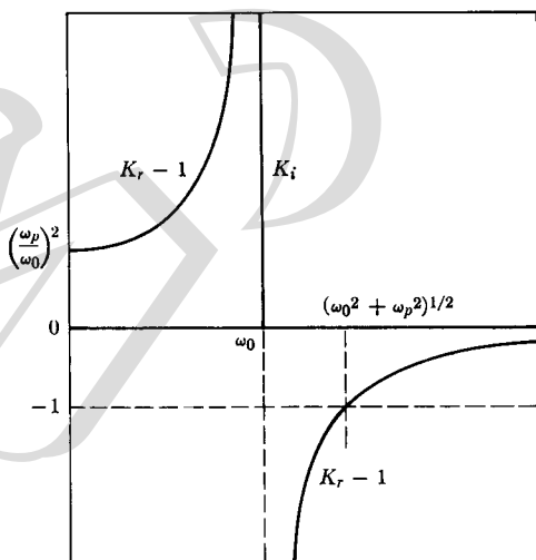
شکل ۱۰۱۹ ثابتهای دی الکتریک بر حسب تابعی از فرکانس برای يك خط جذب بسیار قوی و بسیار باریك
