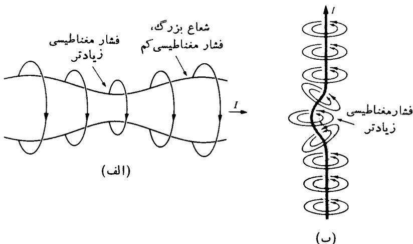
شکل ۷.۱۴ ناپایداریها در پلاسمای تنگیده: (الف) ناپایداری
