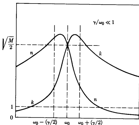
شکل ۴.۱۹ ثابتهای ایتیکی برای يك خط بساریك قوی که از ثابتهای دی الکتريک شکل ۳.۱۹ با M=100 به دست آمده اند. (مبدأ فرکانس در فاصله دور در سمت چپ واقع است.)
