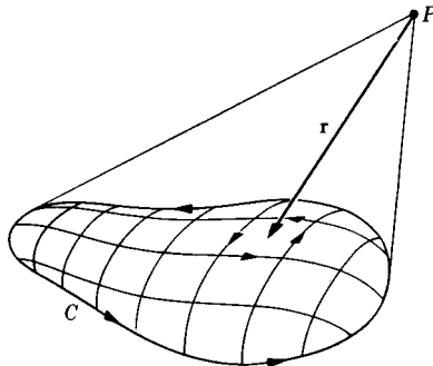
شکل ۱۵۰۸ يك مدار ماکروسکوپی جریان که از عناصر دو قطبی مغناطیسی ساخته شده است.
