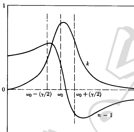
شکل ۵.۱۹. ثابتهای اپتیکی برای یک نوار جذب پهن نسبتاً قوی در \omega_0 .
